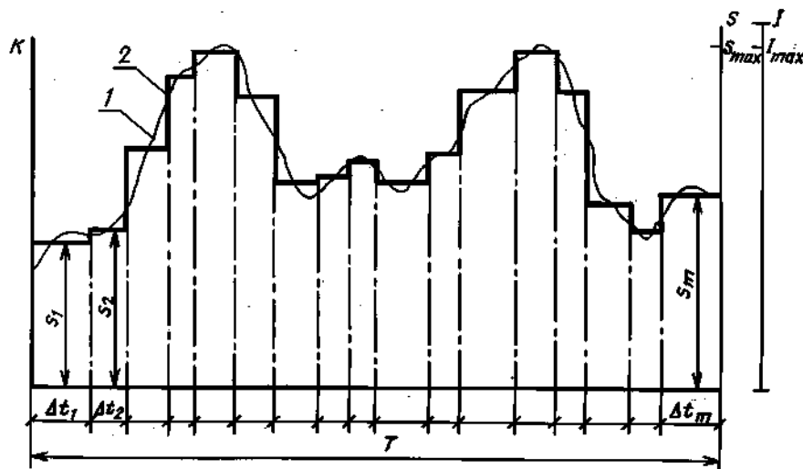
1 — исходный график нагрузки; 2 — эквивалентный прямоугольный график нагрузки
